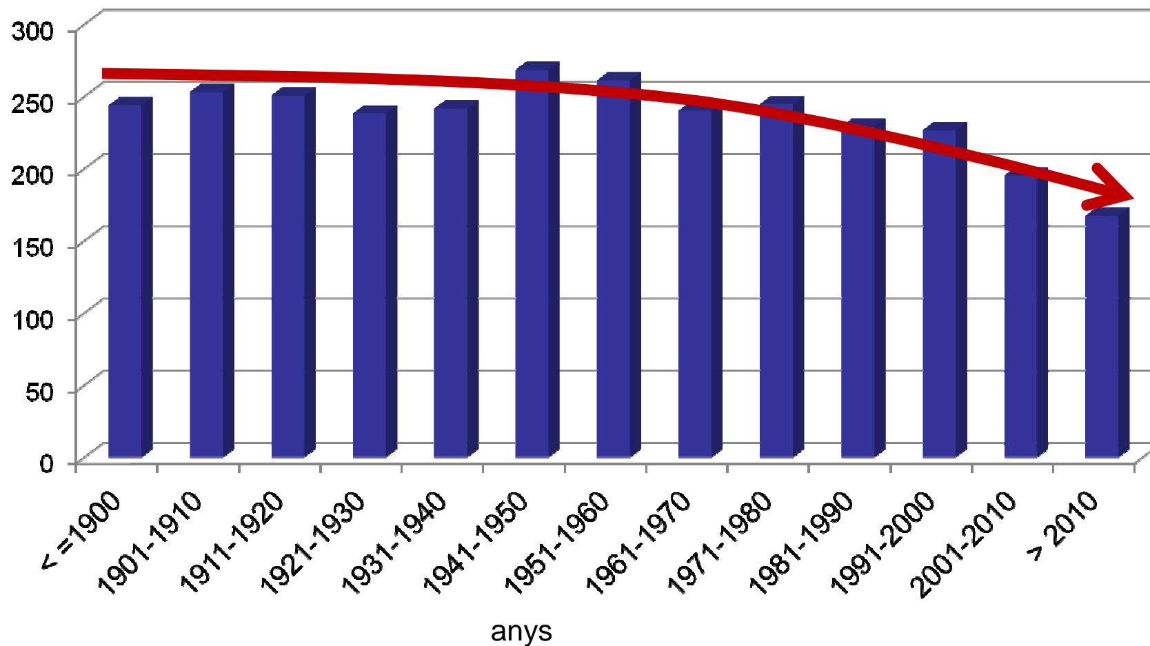
Evolució de la demanda d'energia primària kWh/ m²/ any
